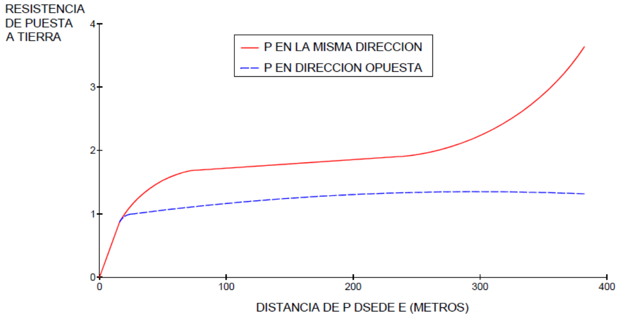
Figura 2, resistencia de puesta a tierra versus distancia de ( \rho )
