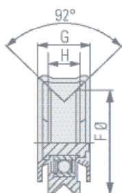
Vista Lateral
